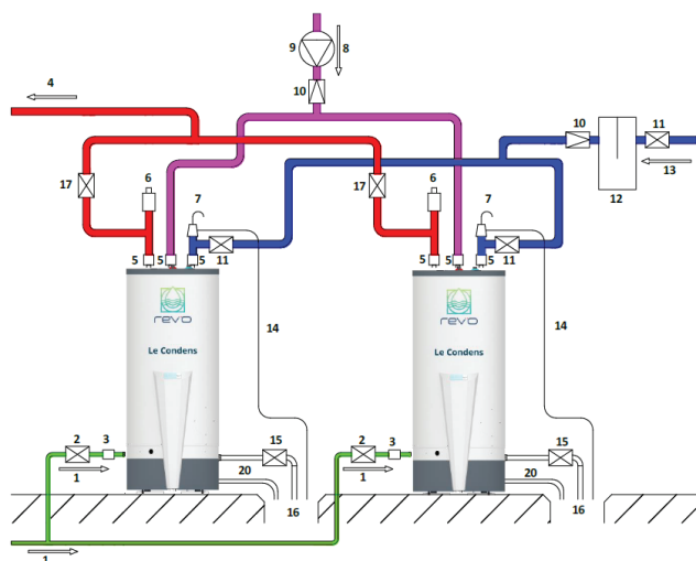
➤ Schéma de principe avec deux accumulateurs en parallèle
