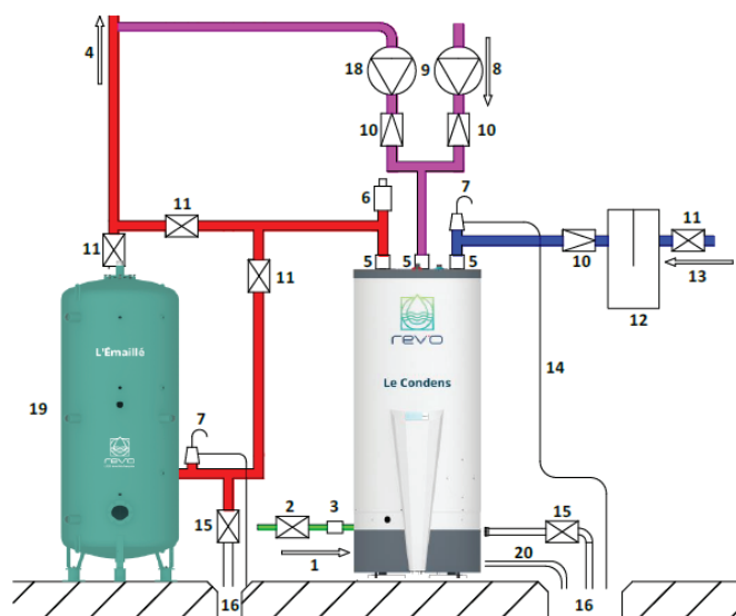
➤ Schéma de principe avec un accumulateur et un réservoir de stockage
