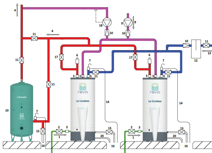
➤ Schéma de principe avec deux accumulateurs et un réservoir de stockage
