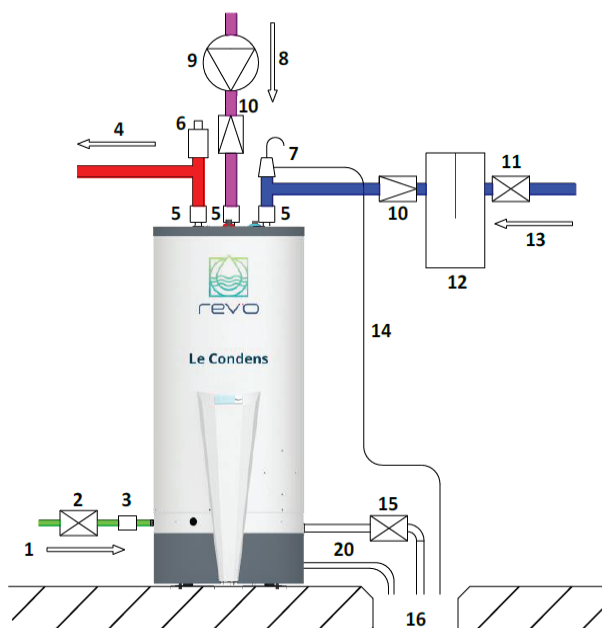
➤ Schéma de principe avec un accumulateur
