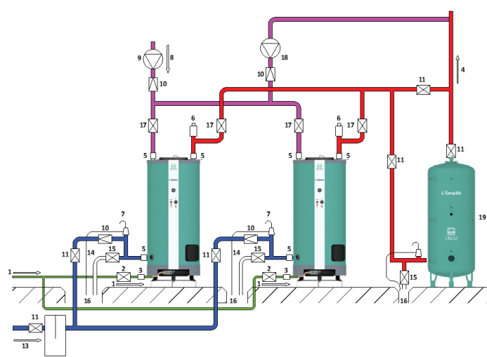
➤ Schéma de principe avec deux accumulateurs et un réservoir de stockage
