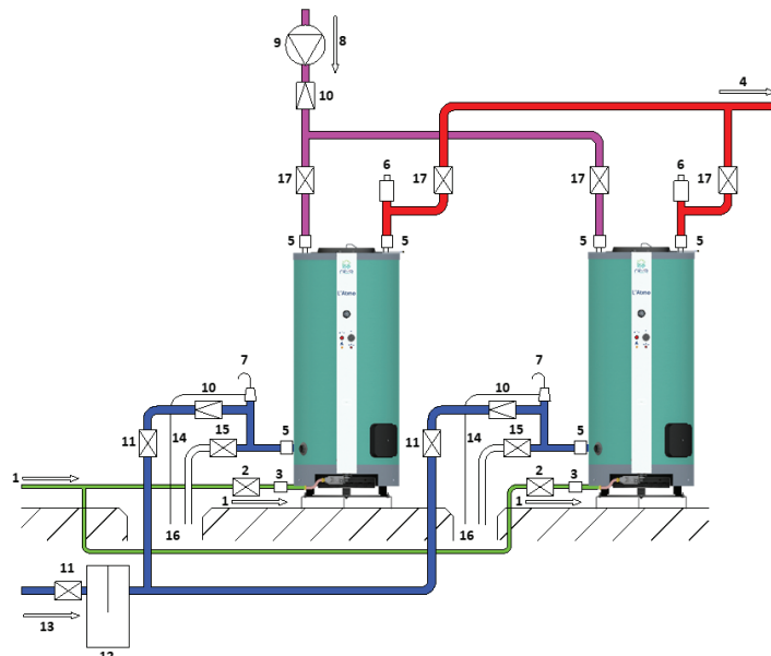
➤ Schéma de principe avec deux accumulateurs en parallèle
