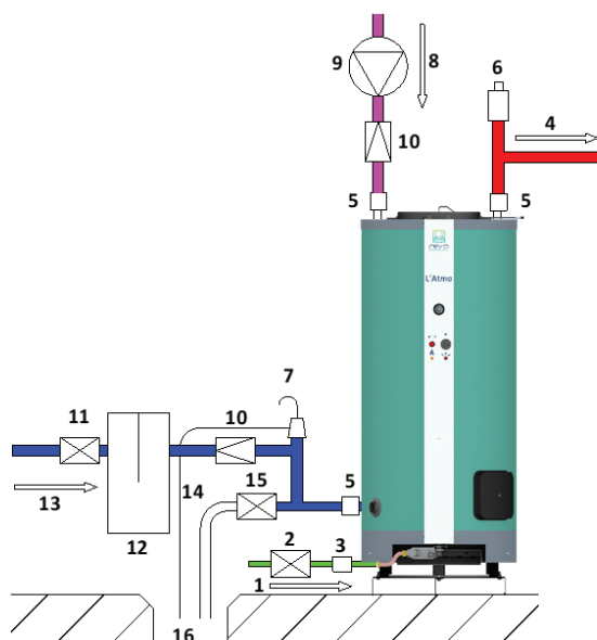
➤ Schéma de principe avec un accumulateur
